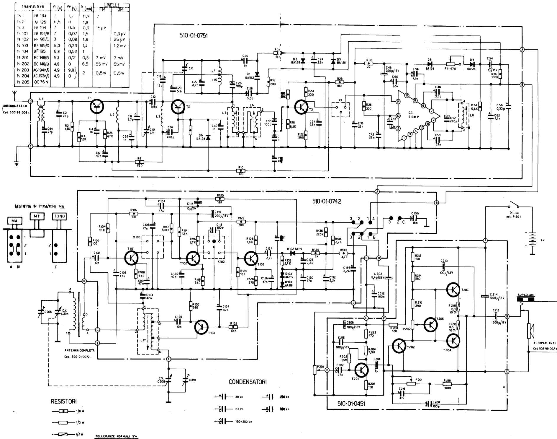
Fig. 9.2 Schema elettrico della radio portatile 15505 V2G della Bruonvega
